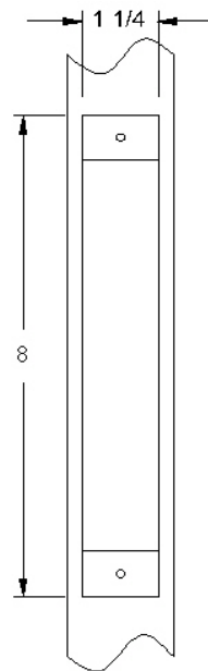
DOOR EDGE MORTISE LOCK PREP ANSI STANDARD A115.1
