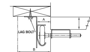
WOOD JAMB
