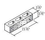
4x4x16 1F HH*
