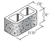
8x8x16 1F, 2E DBN PL*
