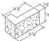
4x8x16 GFE w/ 74° Return
