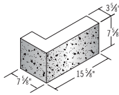
4x8x16 1F, 1E L-Corner
