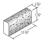
4x8x16 1F, 1T SBN*
