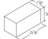
8x8x16 HP Solid
