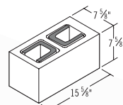
8x8x16 Korfil Insulated*
