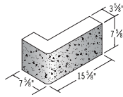
4x8x16 1F, 1E L-Corner SBN
