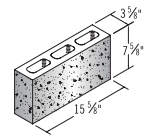
4x8x16 1F, 1E Corner*
