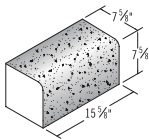
8x8x16 1F, 1T SBN*
