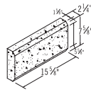
2 1/4 x 8 x 16 GFTE Chamfer
