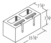
8x8x16 Acousta-Wal Type IV RF
