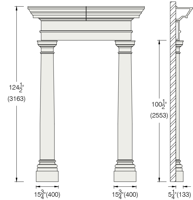
Art Deco Door Surround Retrofit Q340 Tech Sheet: TL46
